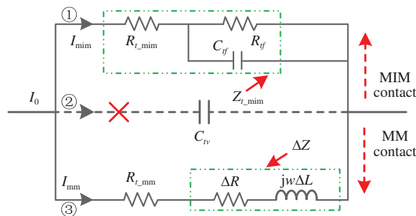
图 9 (网络版彩图) 松散电接触等效电路模型
