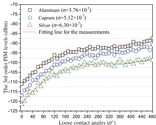
图 11 (网络版彩图) 增加阻抗与三阶无源互调值关系
