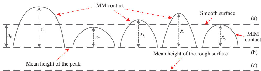
图 6 (网络版彩图) 松散电接触动态模型
