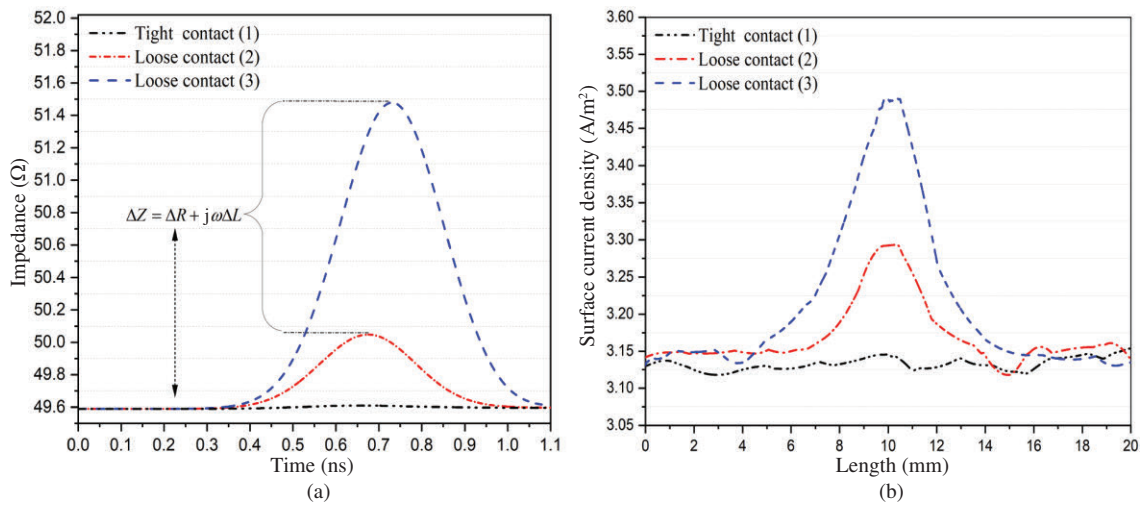
图 8 (网络版彩图) 松散电接触的阻抗与面电流密度仿真. (a) 松散电接触阻抗仿真; (b) 松散电接触面电流仿真
